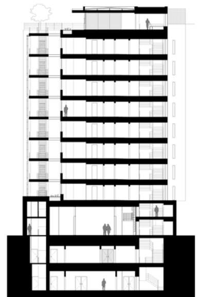
ΤΟΜΗ
