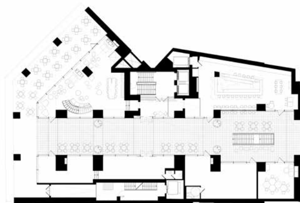
ΚΑΤΩΦΗ ΙΣΟΓΕΙΟΥ
