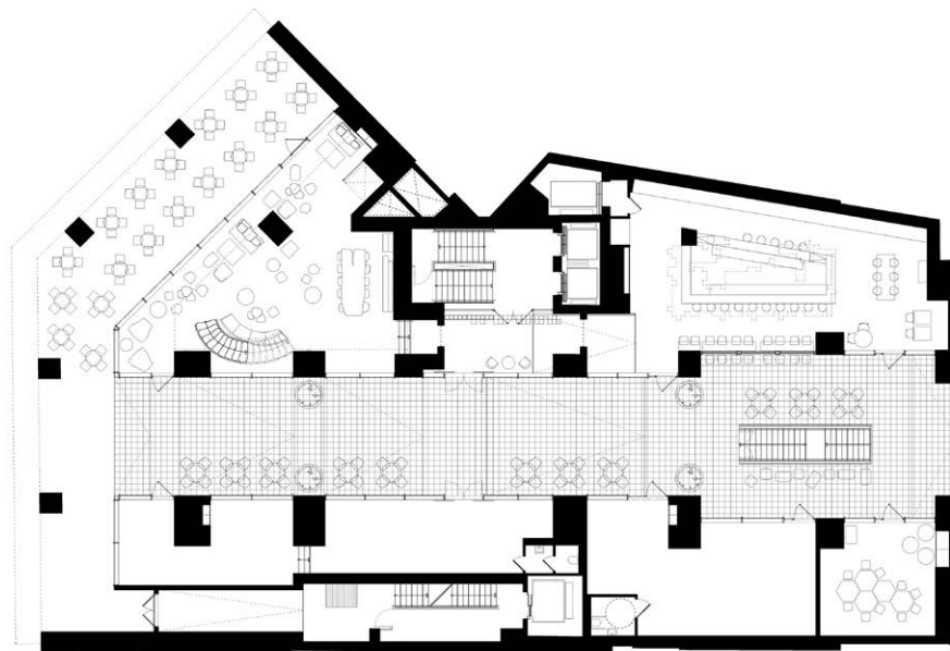
ΚΑΤΩΨΗ ΙΣΟΓΕΙΟΥ
