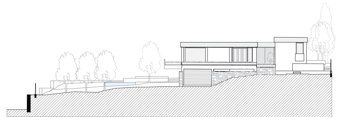
ΝΟΤΙΟΔΥΤΙΚΗ ΟΨΗ
